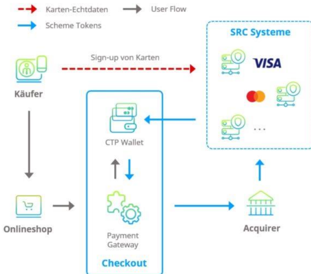
Die Systemarchitektur von Visa Click to Pay. (Grafik: Computop Paygate)
